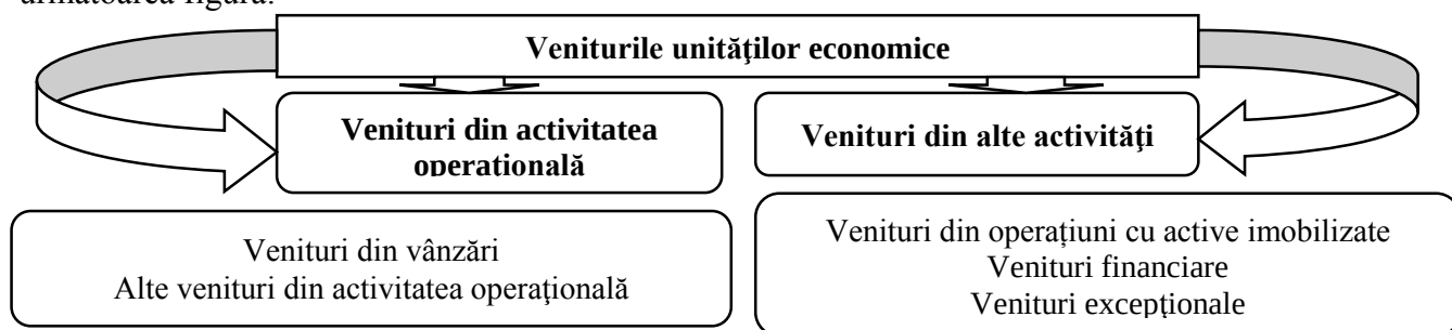
Figura 1. Clasificarea veniturilor
